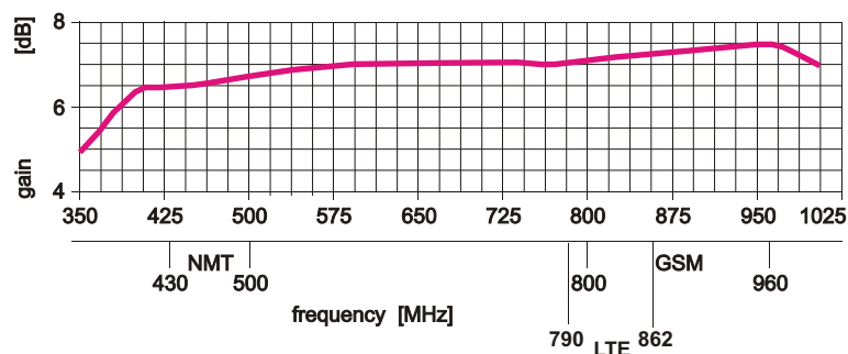
Antennendiagramm
