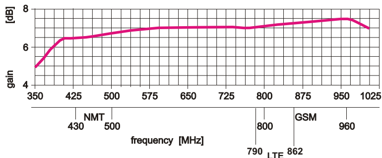
Antennendiagramm
